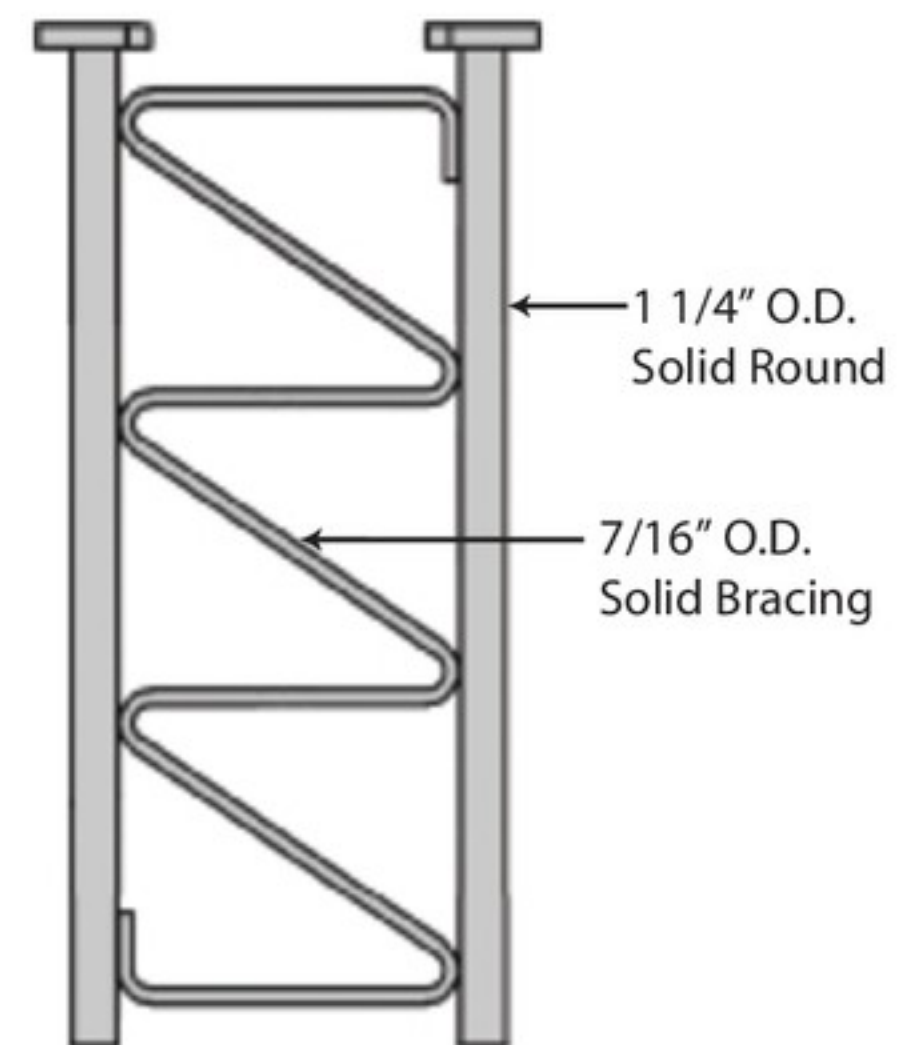
4.3' 45GSR SHORT BASE 45GSRSB
