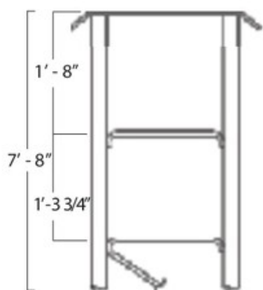
TOP SECTION 45AG4
