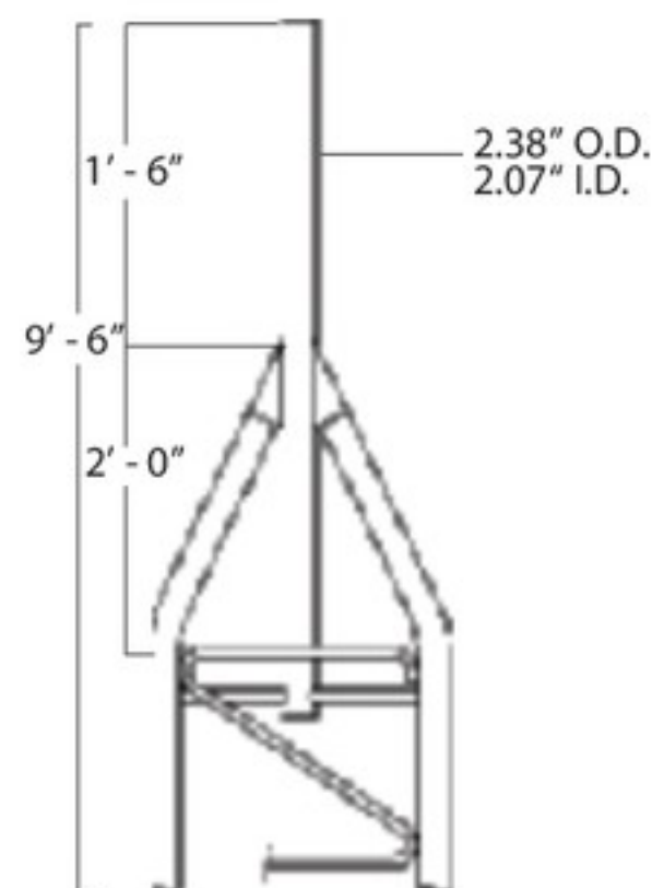
TOP SECTION 45AG2
